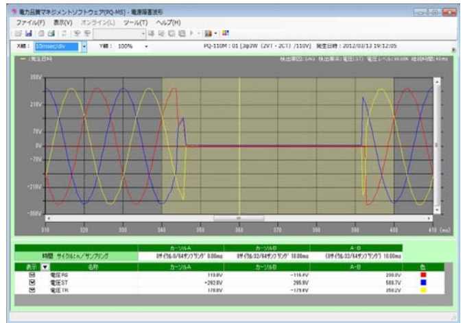
■電源障害波形■
