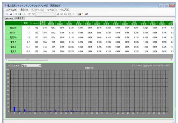
■高調波解析(分析)■
