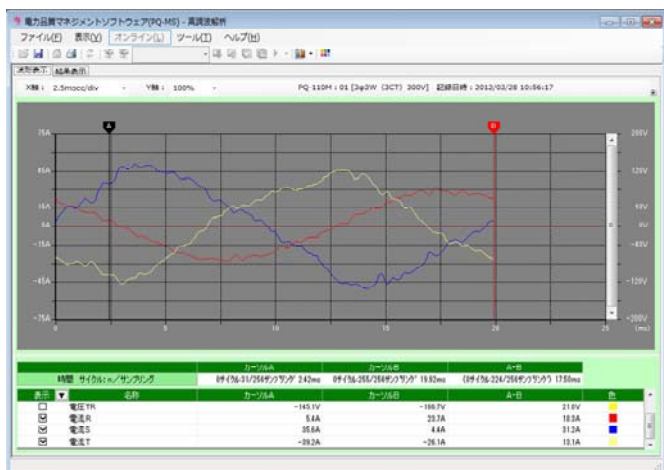
■高調波解析(波形)■
