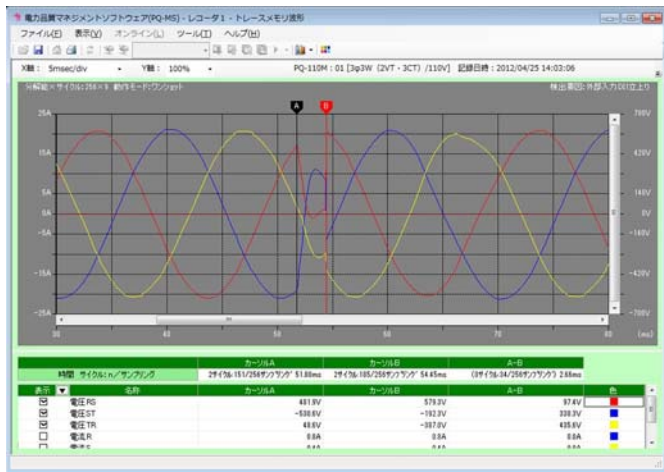
■トレースメモリ波形■
