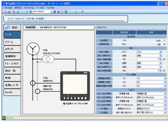
■メータ設定(3φ4W3VT4CT)■
