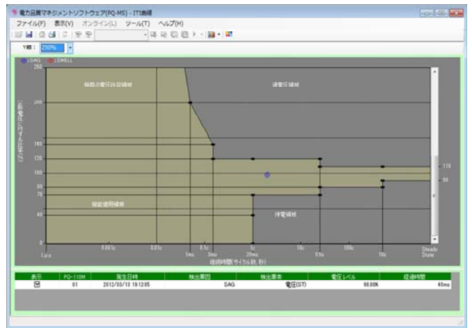
■ITR曲線■
