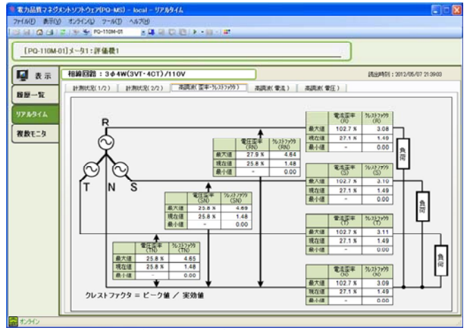
■リアルタイムモニタ(3φ4W3VT4CT)■
